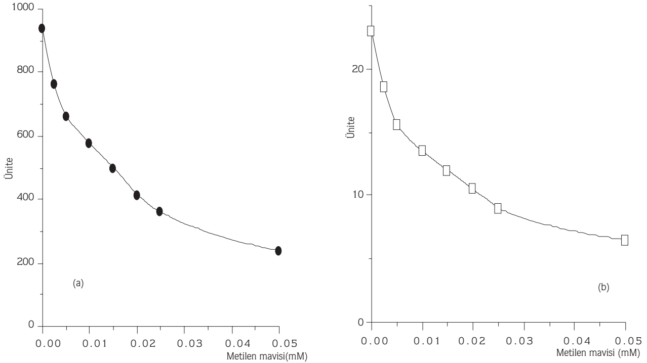
Şekil 1(a-b): Manda karaciğer dokusu(a) ve böbrek dokusu(b) arginazının değişik konsantrasyonlarındaki metilen mavisi ile fotoinaktivasyon eğrisi.
